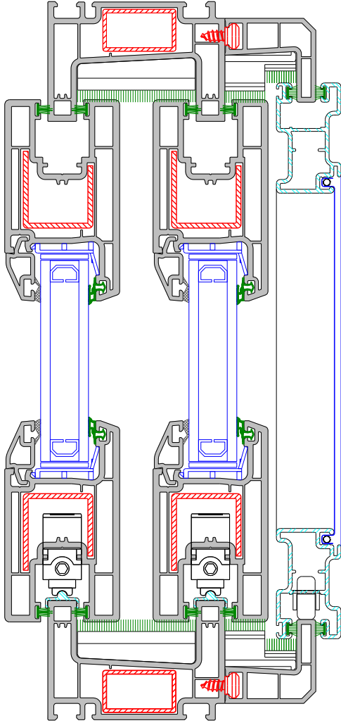
A-A
